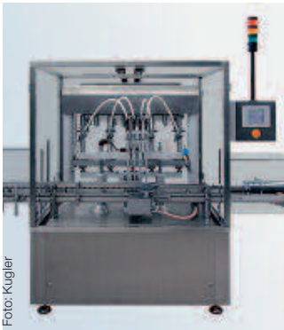
Concepto modular de máquina para productos líquidos hasta pastosos.
